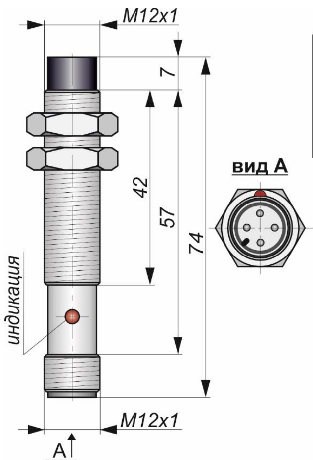
Габаритный чертеж
