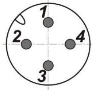
Цоколевка разъема
